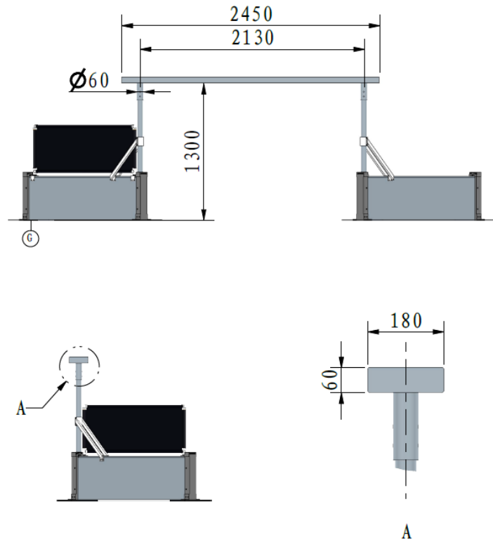
图 3-6 哨兵轨道示意图
