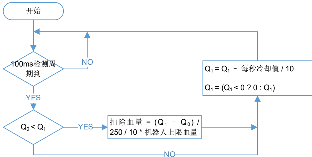
图 2-2 枪口热量超限的扣血逻辑图（上）和冷却逻辑图（下）
