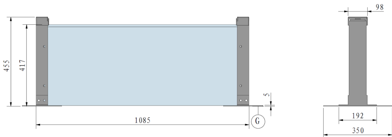
图 4-4 掩体示意图
